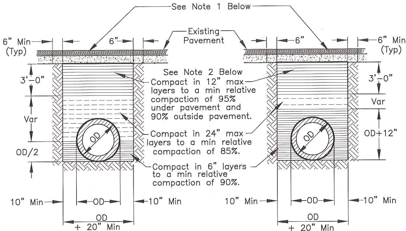
FLEXIBLE CONDUIT
